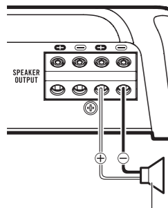
Lautsprecherausgang
