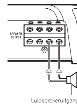
Luidsprekeruitgang
