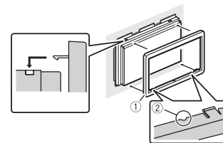
1 Moldura 2 Orifício Coloque a moldura com a ranhura apontada para baixo.
