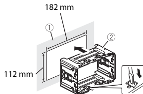
① Salpicadero
