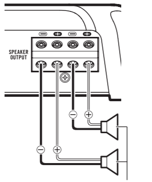
Lautsprecherausgang
