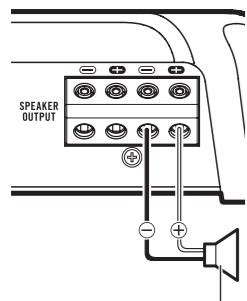
Lautsprecherausgang
