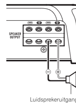
Luidsprekeruitgang
