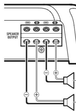
Luidsprekeruitgang
