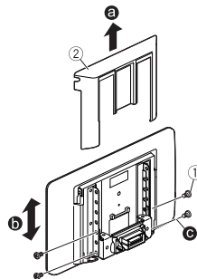
① Vis de fixation (4 mm × 6 mm) ② Couvercle du moniteur
