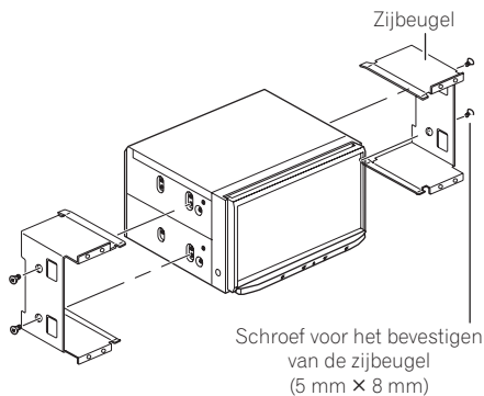
Zijbeugel
