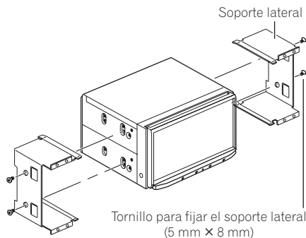
Soporte lateral
