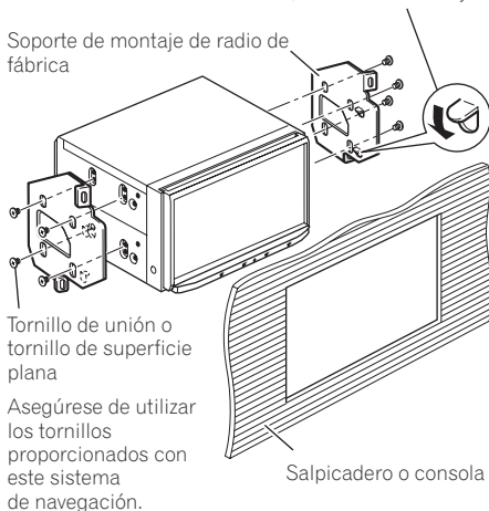
Soporte lateral
