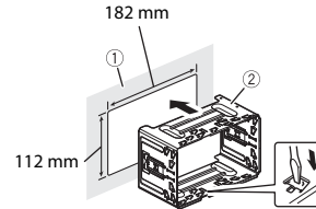
① Salpicadero ② Soporte
