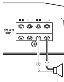
Выход громкоговорителя
