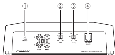
Face arrière
