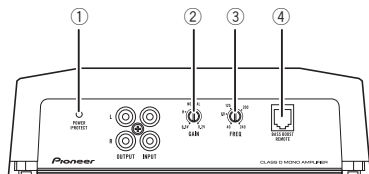
Parte trasera
