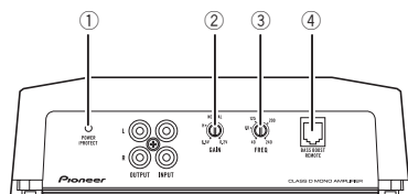
Face arrière
