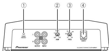
Задняя панель
