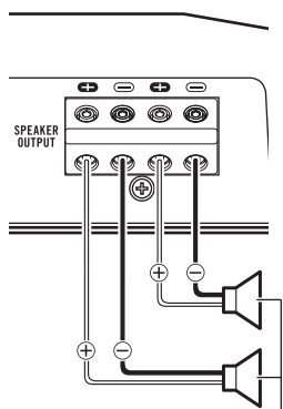
Выход громкоговорителя
