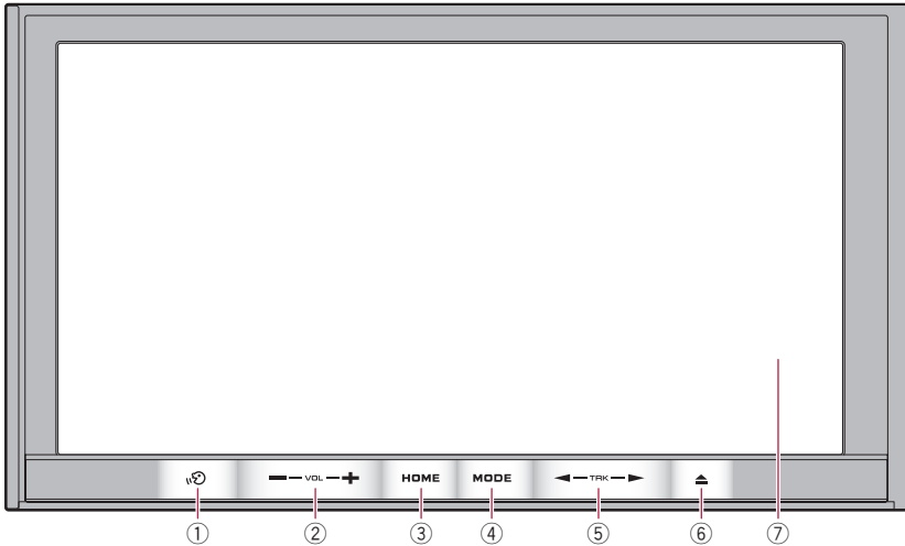
AVIC-F20BT (mit geschlossener LCD-Tafel)
